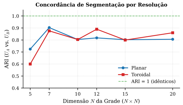
Figura 3. Adjusted Rand Index (ARI) entre segmentações U_A e U_B por dimensão de grade N .
