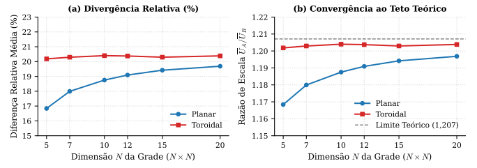
Figura 2. Sistemática da divergência vs. dimensão N : (a) Divergência relativa (%); (b) Razão de escala \bar{U}_A/\bar{U}_B e teto teórico 1,207.
