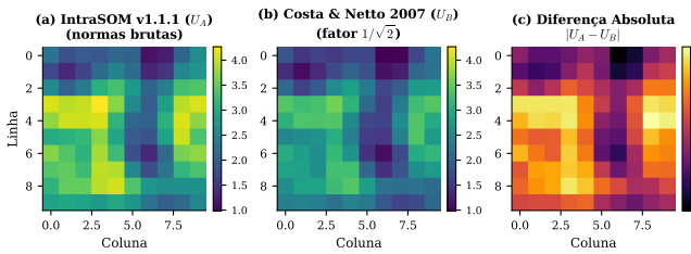
Figura 1. Comparação das U-matrizes U_A (IntraSOM v1.1.1) e U_B (Costa & Netto 2007) para SOM 10 \times 10 RECT toroidal: (a) U_A sem normalização; (b) U_B com 1/\sqrt{2} ; (c) |U_A - U_B| .
