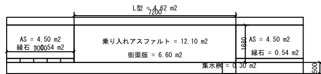
10t用乗入図
