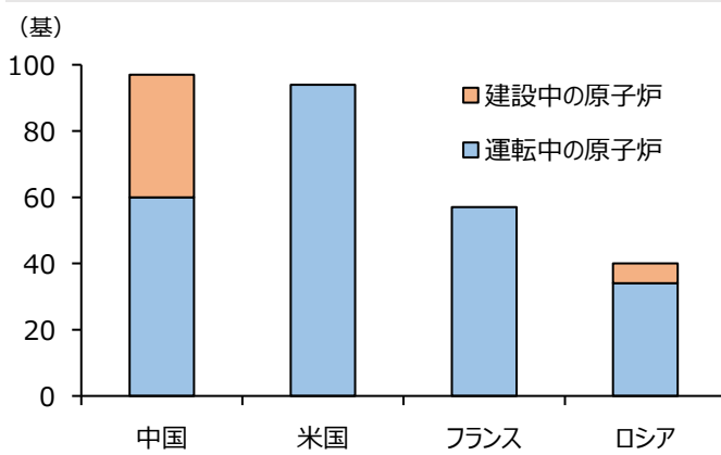
各国で運転中と建設中の原子炉の数
