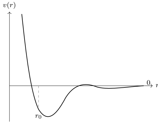
図 2 典型的な二体ポテンシャル v(r) .
