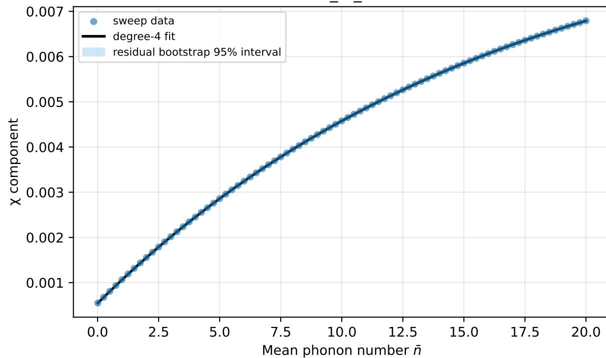
chi_XI_XI
