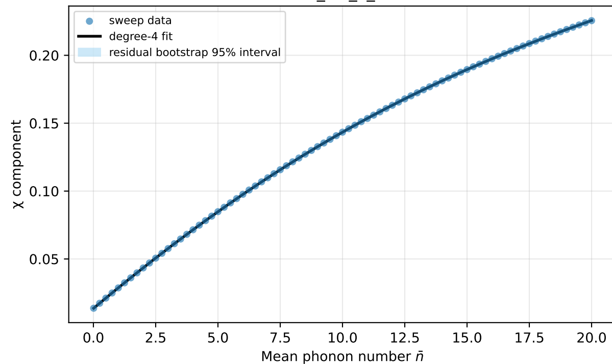
abs_chi_II_XX
