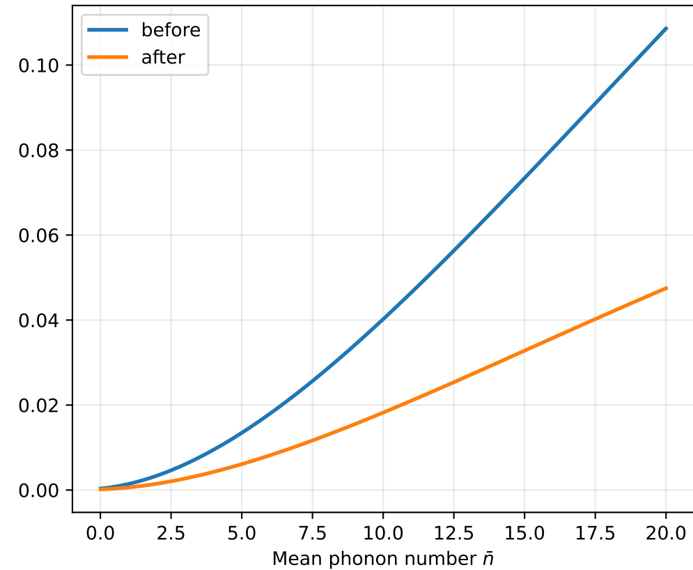
\chi_{XX,XX}
