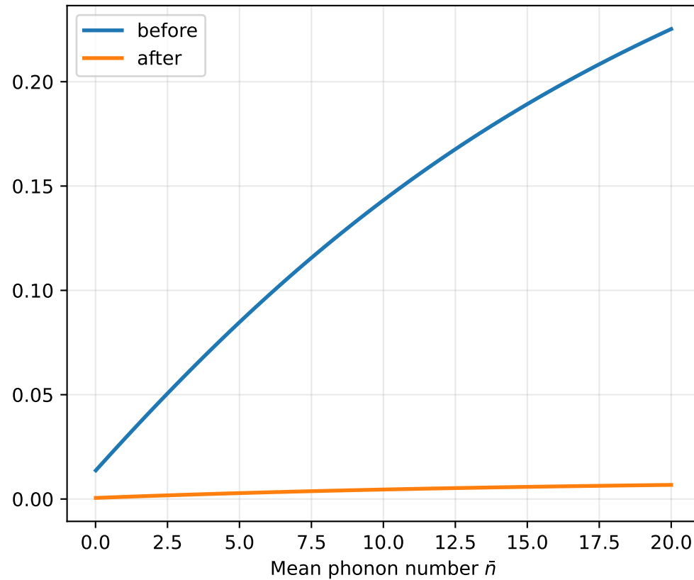
|\chi_{II,XX}|
