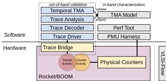
Fig. 4: Icicle overview.
