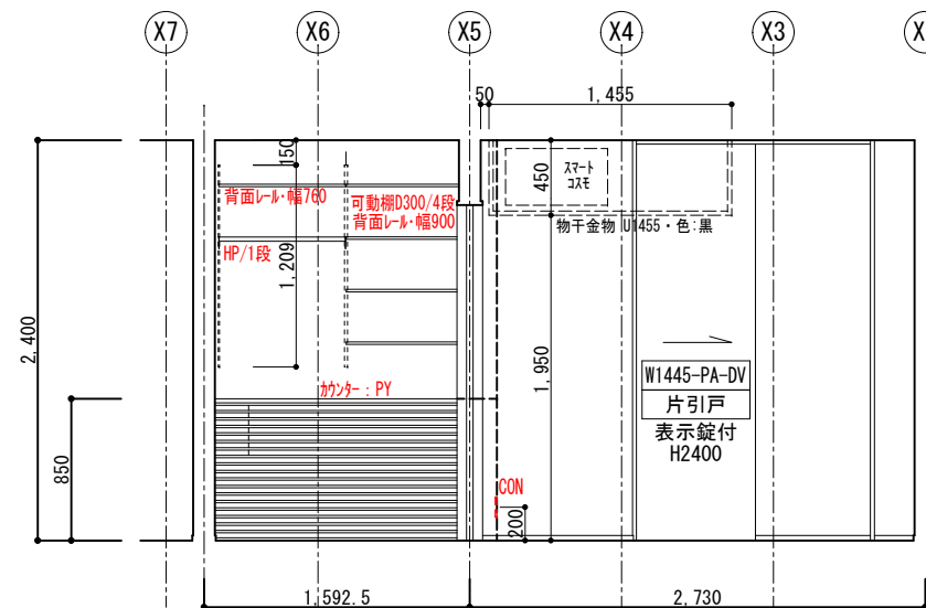
【脱衣所・ランドリールーム C展開図 1/50】
