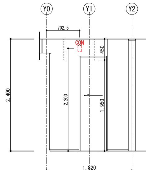
【LDK D展開図 1/50】
