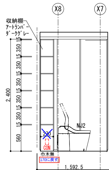
【トイレ D展開図 1/50】
