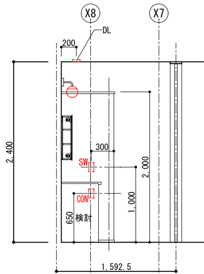
【洗面コーナーC展開図 1/50】
