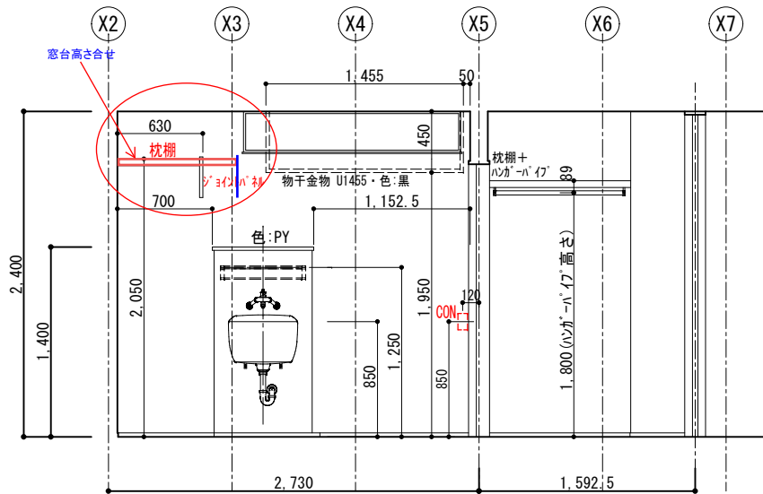
【脱衣所・ランドリールーム A展開図 1/50】
