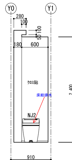
【トイレ B展開図 1/50】
