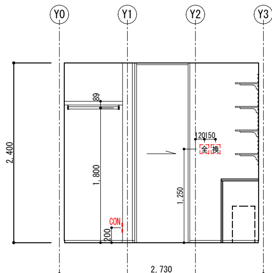
【脱衣所・ランドリールーム D展開図 1/50】
