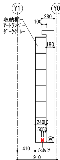
【トイレ C展開図 1/50】
