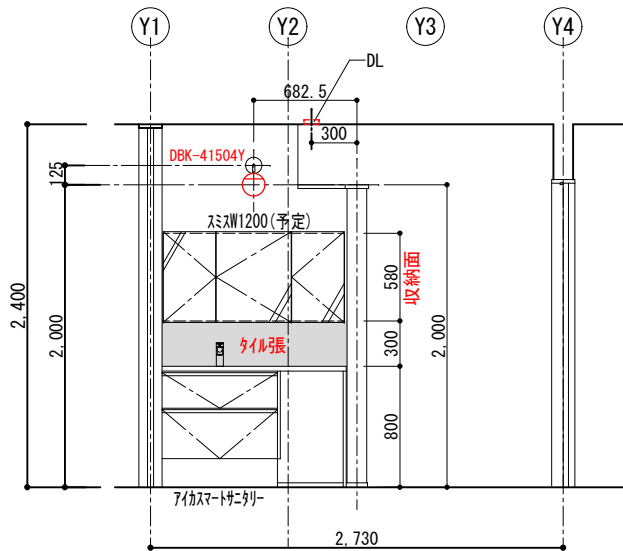
【洗面コーナーB展開図 1/50】
