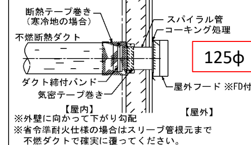
サイクロン式給気フード詳細図
