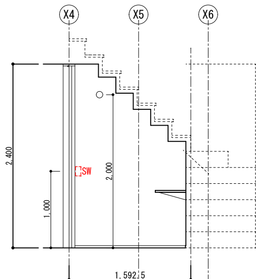
【階段下収納 A展開図 1/50】
