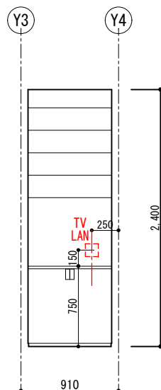
【階段下収納 B展開図 1/50】
