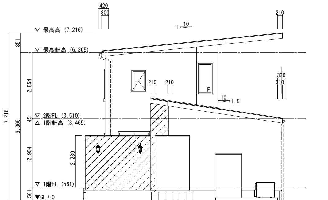
東側立面図
