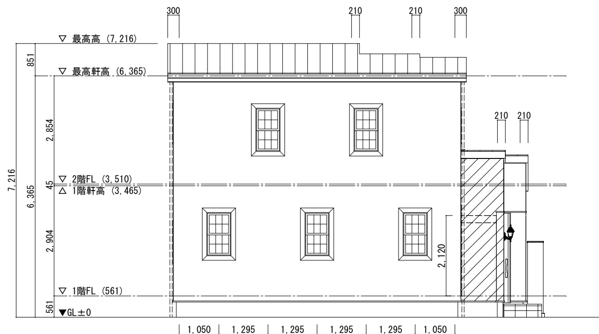
南側立面図
