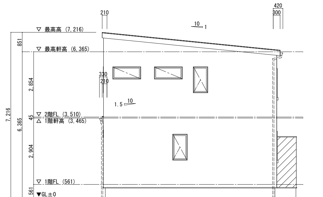
西側立面図
