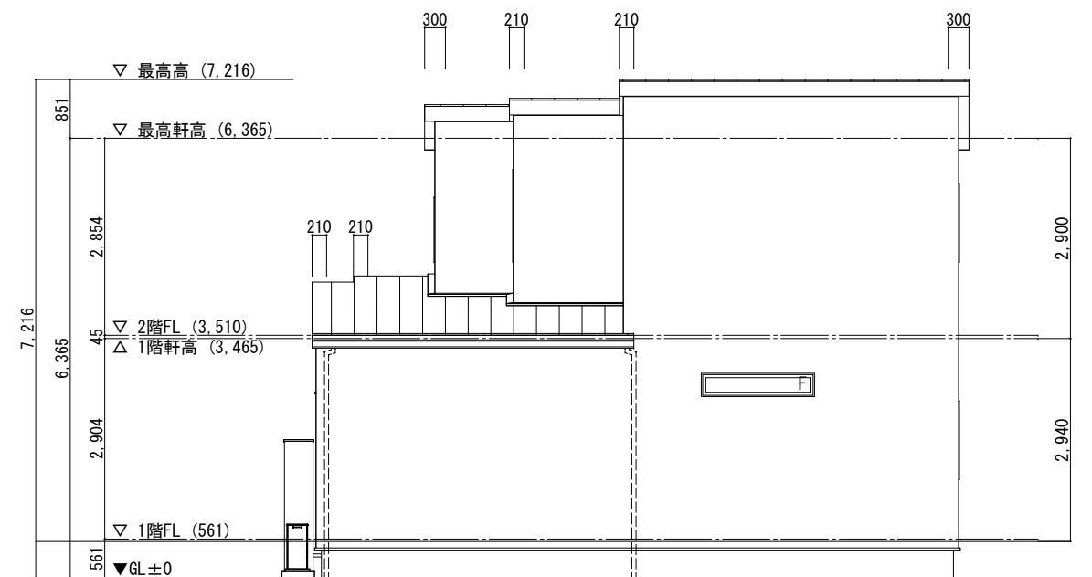
北側立面図
