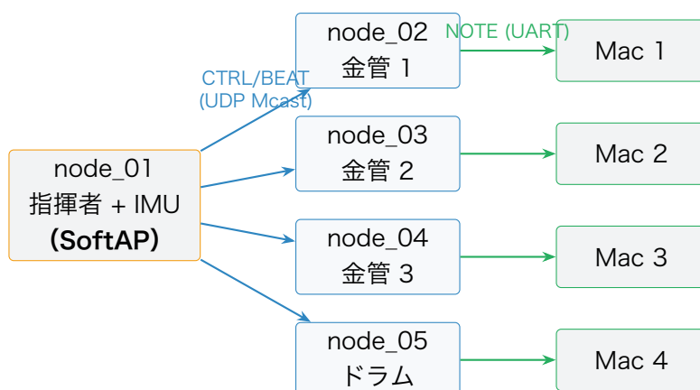
図 2.1 全体ブロック図（指揮者 node_01 が SoftAP を兼ね、楽器 4 台が STA 接続。楽器 → Mac は 1 対 1 USB Serial）
