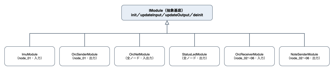
図 3.1 モジュールのクラス継承関係 (各モジュールの所属ノードを併記)
