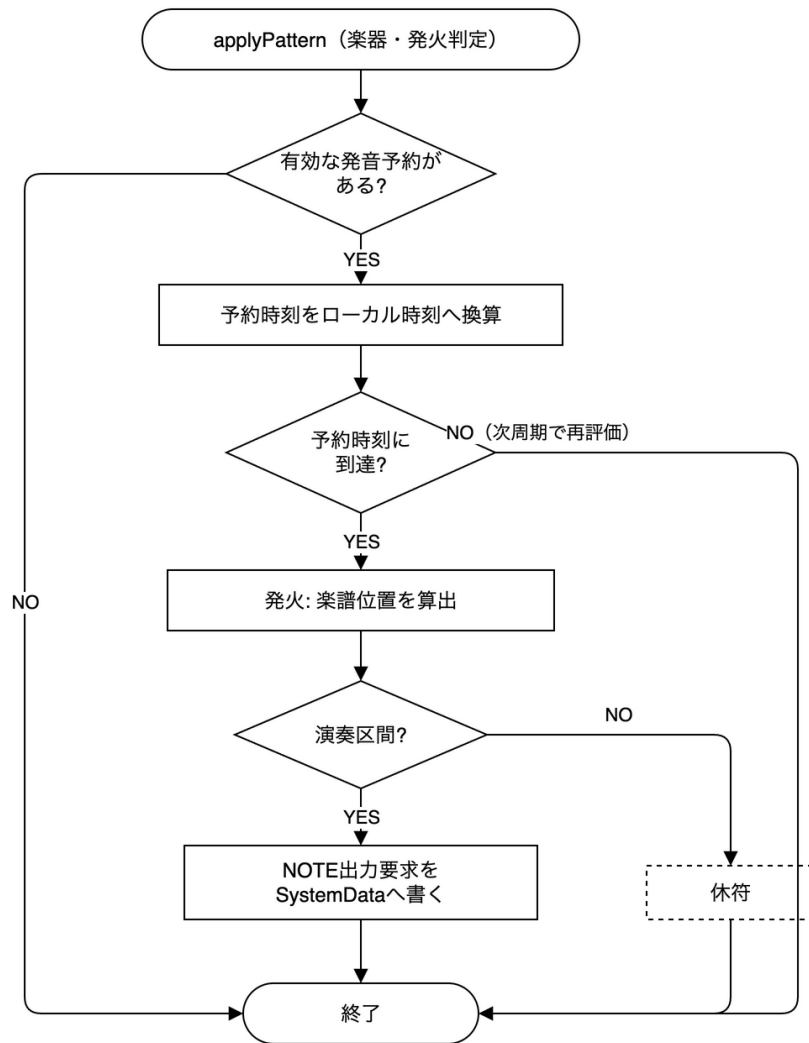
図 A.22 applyPattern() 関数（楽器：発音予約の発火・楽譜進行）のフローチャート
