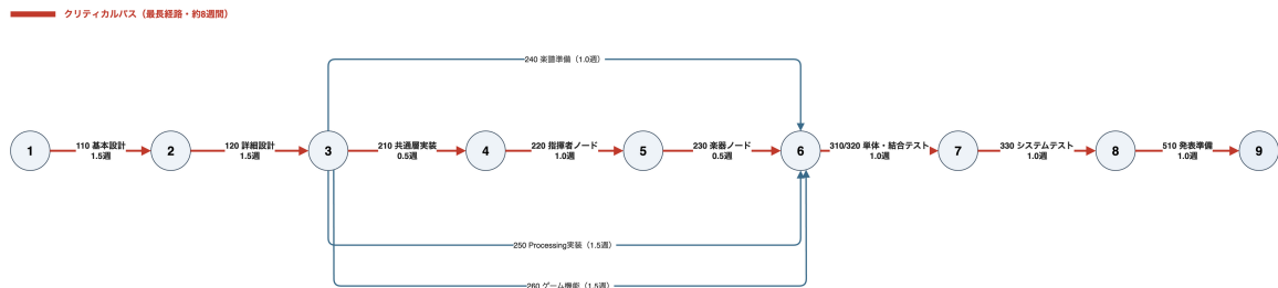
図 1.3 アローダイアグラムとクリティカルパス
