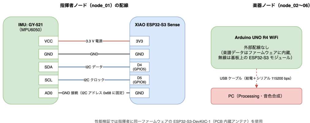
図7 ハードウェア構成 (左: 指揮者ノードの配線, 右: 楽器ノードと PC の接続)
