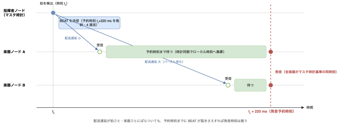
図 3 発音予約と時計同期による同期の原理（配送遅延のばらつきを待ち時間が吸収する）
