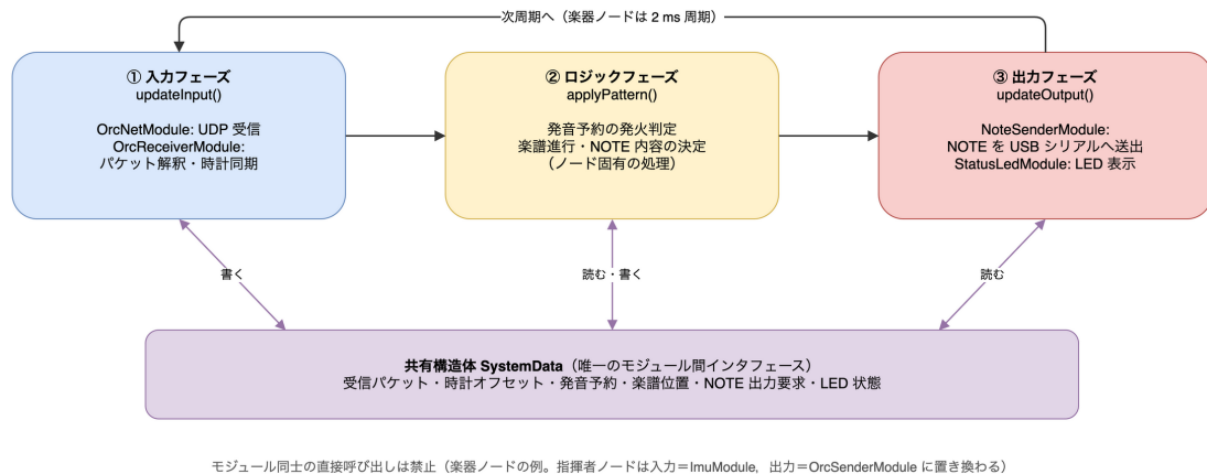
図 4 Embedded-Module-Architecture の 3 フェーズループと共有構造体
