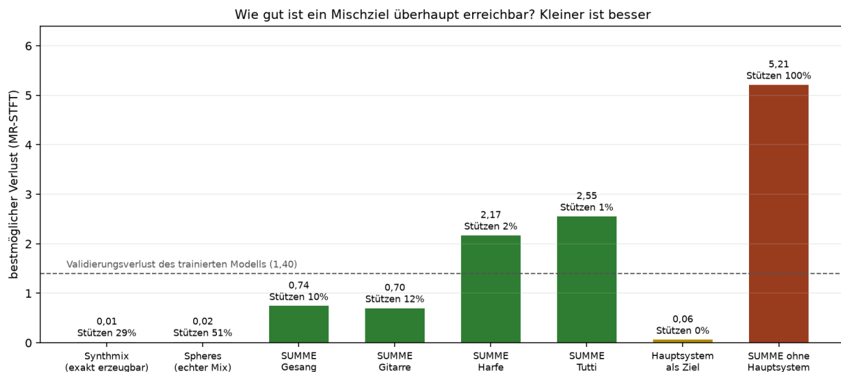
Abbildung 7: Bestmöglicher Verlust je Ziel, gemessen in der Trainings-Verlustfunktion. „Stützen“ ist der Energieanteil der Stützmicrofone in der optimalen Mischung: Er sagt, wie viel über sie überhaupt zu lernen wäre.
