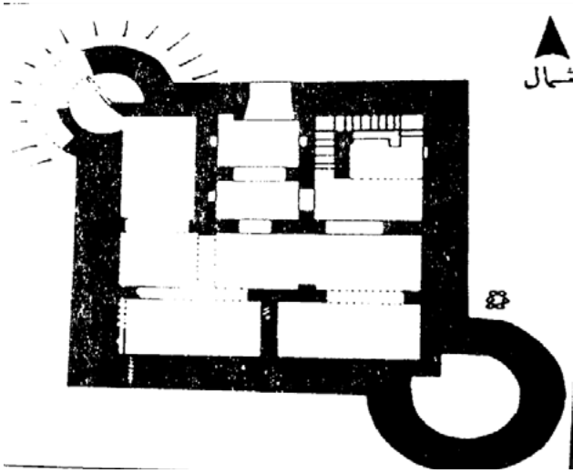
(شكل ١٢) التخطيط المعماري لحصن النعمان/ الباطنة/ نقلا عن (القلاع والحصون)
