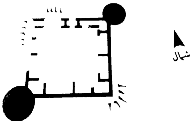
(شكل ١٤) التخطيط المعماري لحصن البو خميس/ الباطنة/ (نقلا عن القلاع والحصون)
