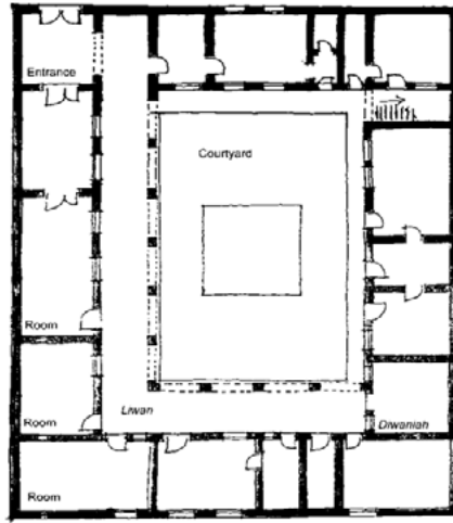
(شكل ٢٥) الشكل العام لتخطيط المنزل الكويتي القديم
