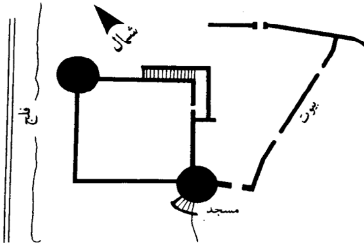
(شكل ١٣) التخطيط المعماري لحصن أفي / الغاف/ (نقلا عن القلاع والحصون)
