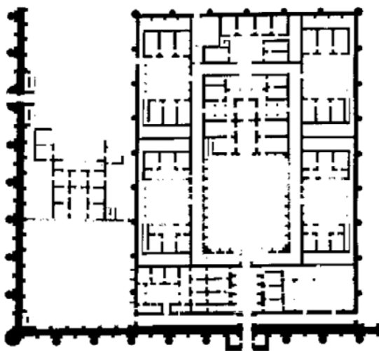
(شكل ٢٤) المخطط المعماري بقصر الأخيضر العباسي
