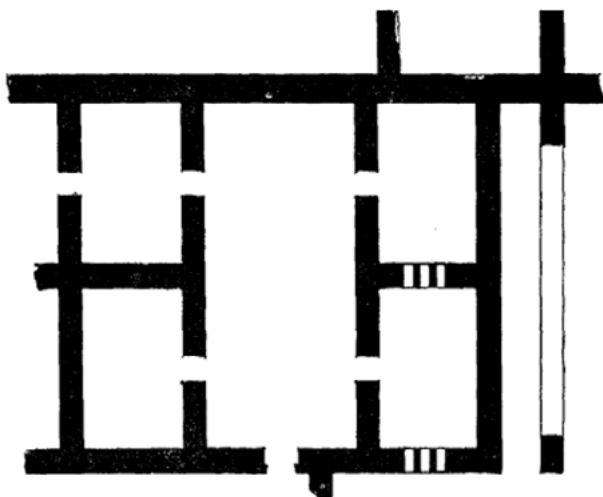
(شكل ١٩) قصر الطوبة - نموذج مسكن - نقلا عن فريد شافعي
