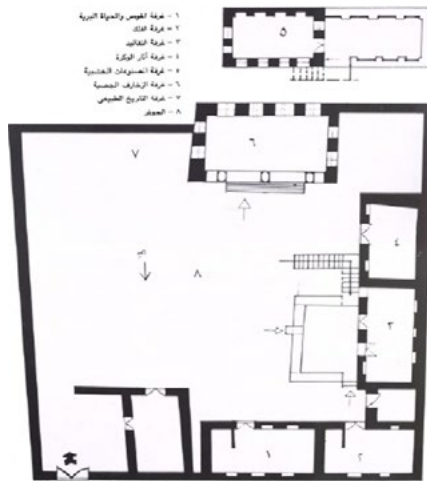
(شكل ٢٦) دار عبد الله بن سعد بمدينة ألوك
