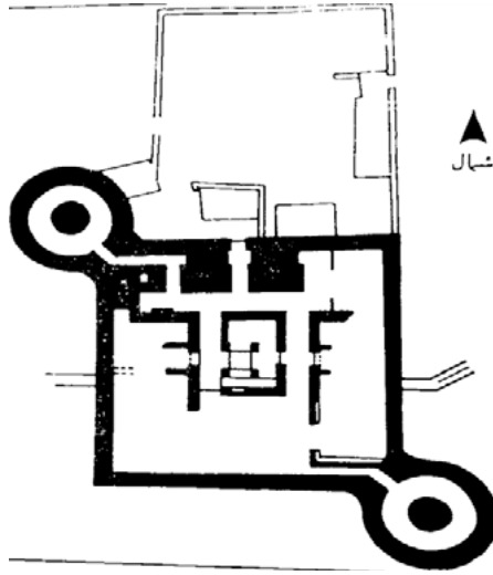
(شكل ٤) التخطيط المعماري لحصن الحزم/ الباطنة/ نقلا عن القلاع والحصون.
