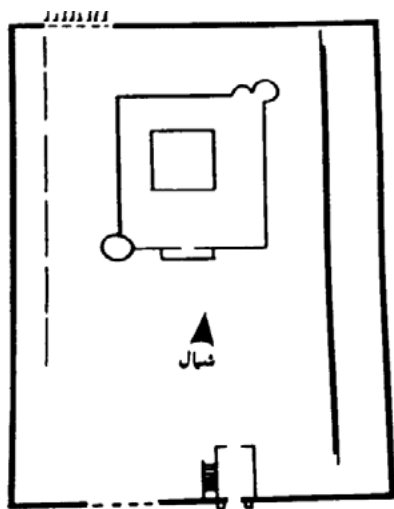
(شكل ١٠) التخطيط المعماري لحصن بركة الموز (بيت رديدة) (نقلا عن القلاع والحصون)
