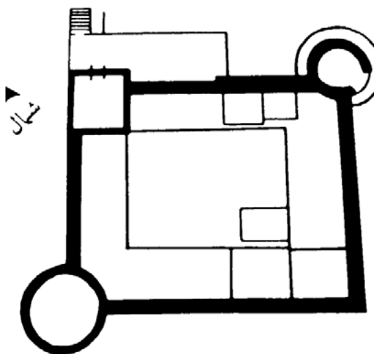
(شكل ١٥) التخطيط المعماري لحصن العوابي/ الباطنة/ نقلا عن (القلاع والحصون)
