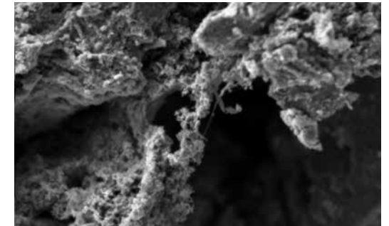
在高放大倍率和低加速电压下对催化剂颗粒成像（左：钨灯丝，右：六硼化镧）。在高难度成像条件下，用户可以利用六硼化镧点光源高达 10 倍的束流亮度来增强图像分辨率和衬度。水平观察视野：20 μm。
