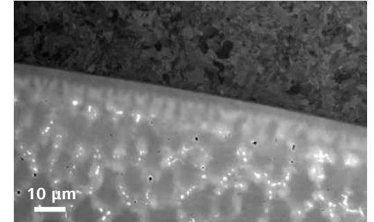
在蔡司 EVO 15 下使用 BSD 探测器查看 8630 钢上的合金 625 堆焊。样品由 TWI Ltd. 提供。
