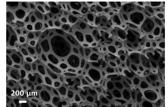
在可变压力模式下，使用 BSE 探测器对汽车座垫泡沫进行无导电涂层成像。
