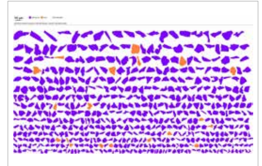
重矿物砂料的颗粒图像，采用费雷特（Feret）最大直径法分选。
