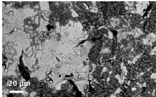
低碳钢腐蚀区域，在蔡司 EVO 15 下使用 BSE 探测器成像。
