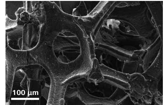
在高真空中使用 SE 探测器对电池装配配件中的泡沫石墨烯结构成像。
