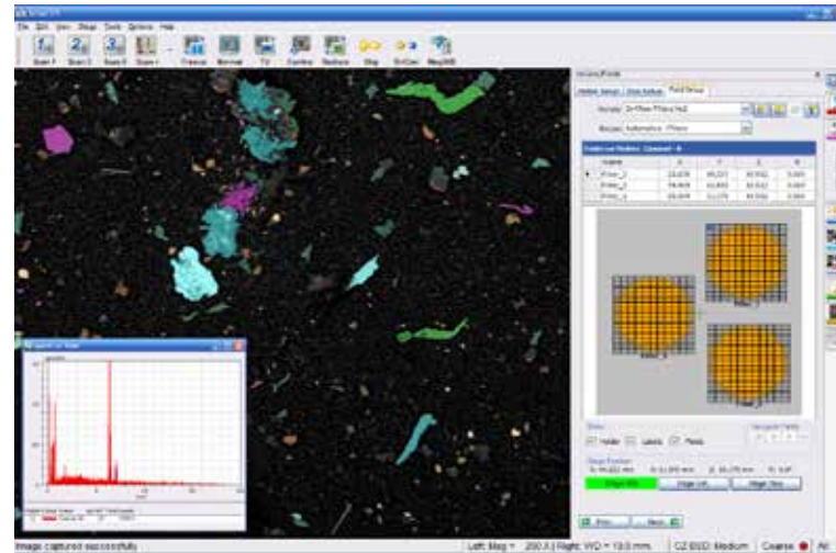
SmartPI 和 EDS：快速颗粒辨识和分类。
