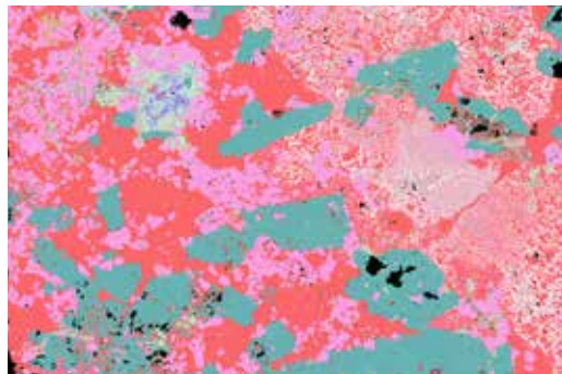
加拿大魁北克过碱性花岗岩，含稀土元素，包括横切样品和分区锆石的萤石矿。
