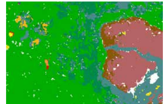
富含 PGE 的豆荚状铬铁勘探物的高分辨率图像。图片由 Chris Brough 博士和威尔士 University of Cardiff 大学提供。
