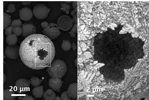
在高真空下使用双放大倍率采集到的钪铁颗粒二次电子图像。
