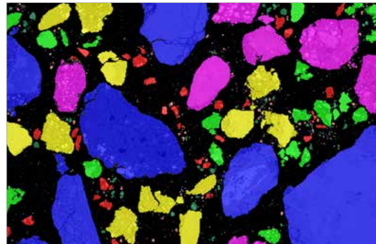
使用蔡司 SmartPI 工具成像，以不同颜色表征大小不同的颗粒。使用 SmartPI 自动定位和表征颗粒，然后再运用图像分析和 EDS 进行标识。数据库中的颗粒目录及全套补充多模式数据 - 随时可供评估和报告使用。
