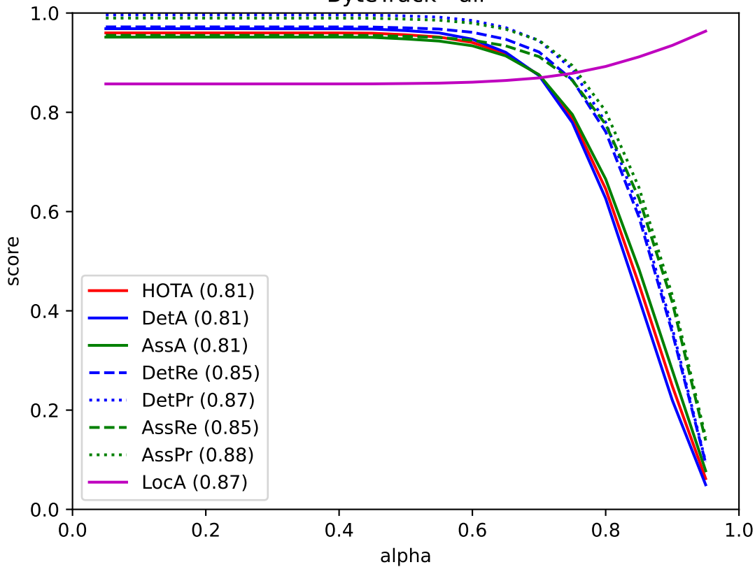
ByteTrack - all
