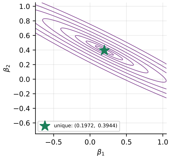
\lambda = 1 : contours CLOSE eigenvalues (1, 71)
