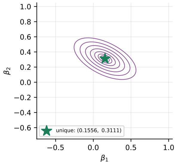
\lambda = 20 : contours CLOSE eigenvalues (20, 90)
