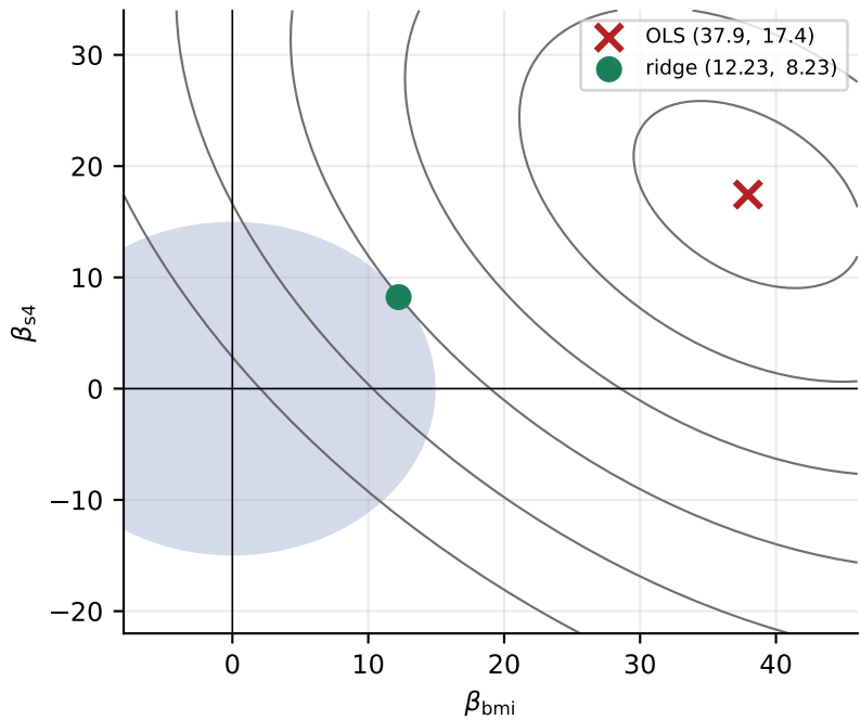
\|\beta\|_2 \leq s : a disc, no corners
