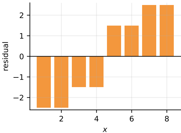
residuals y - F_0
