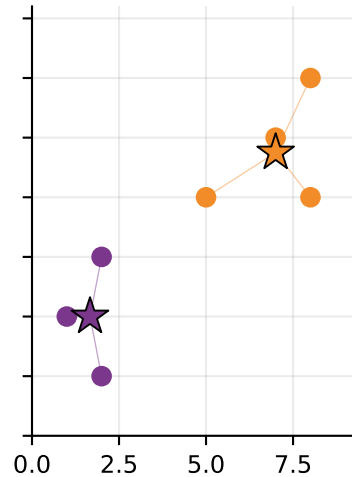
4. update WCSS = 11.4167
