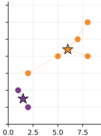
2. update WCSS = 32.2000
