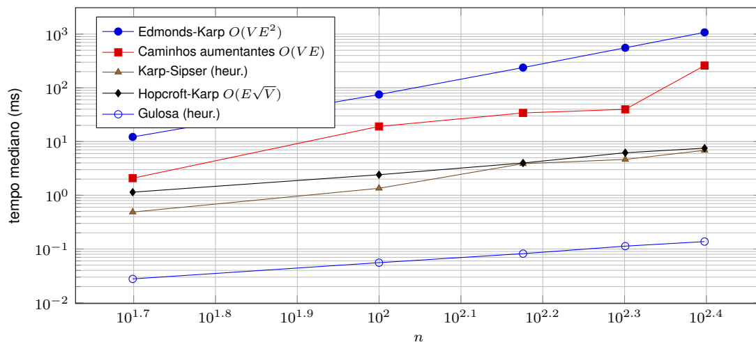
Figura 1: Tempo de execução em escala log-log para o grafo denso (cardinalidade máxima bipartida). A inclinação de cada reta corresponde ao expoente empírico de crescimento; a de Edmonds-Karp, próxima de 3, destaca-se das demais.
