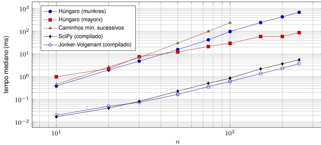
Figura 2: Tempo de execução em escala log-log para a matriz densa (atribuição linear). As duas implementações de núcleo compilado situam-se bem abaixo das interpretadas, mas com inclinação semelhante.
