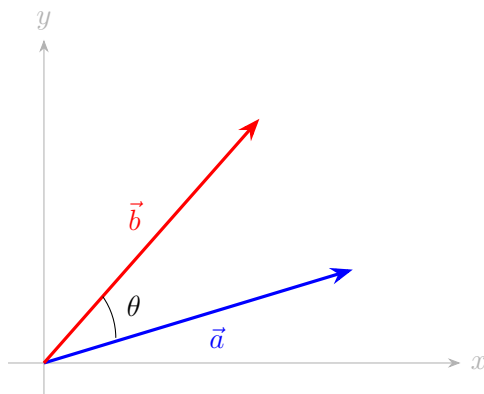
2つのベクトルのなす角 \theta
