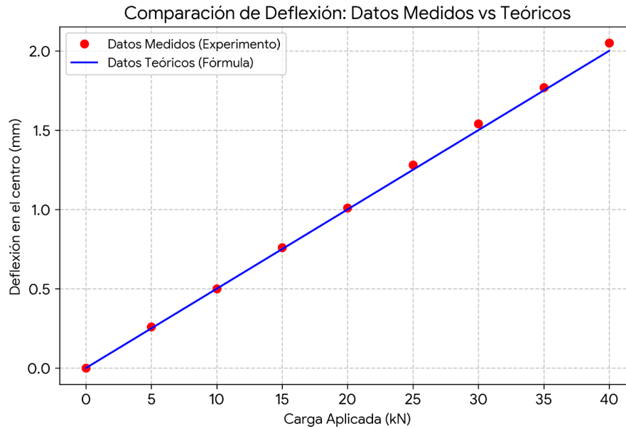
Figura 1: Comparación de deflexión: Datos medidos vs Datos teóricos.
