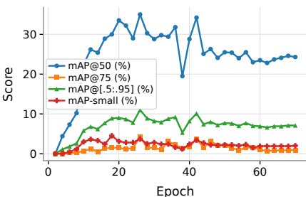
(g) ATSS R50
