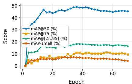
(j) RTMDet-m
