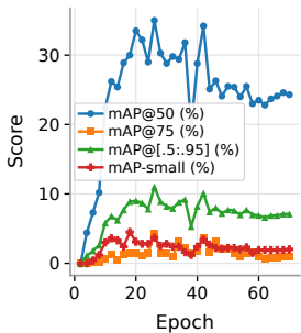
(g) ATSS R50
