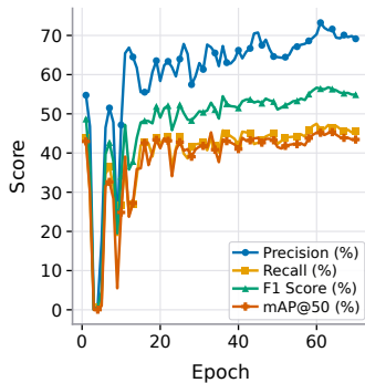
(f) YOLO11m
