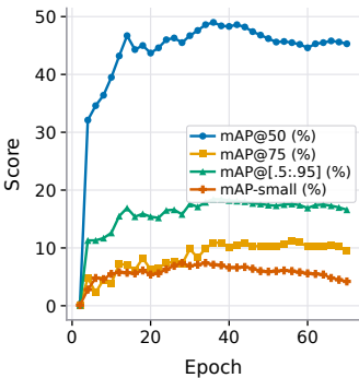
(e) RTMDet-m
