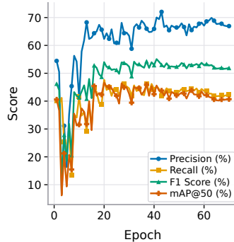
(d) YOLOv9m
