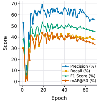
(c) YOLO12m
