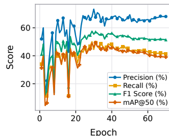
(g) YOLOv9m @1280
