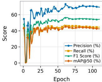
(b) YOLO11m
