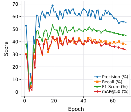
(c) YOLO12m
