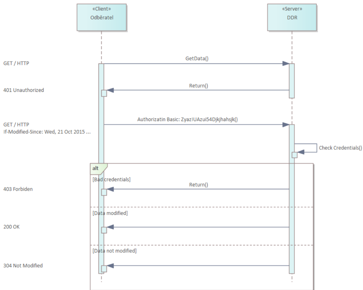
Obrázek 3 Princip komunikace GET Basic Authentication If-Modified-Since
