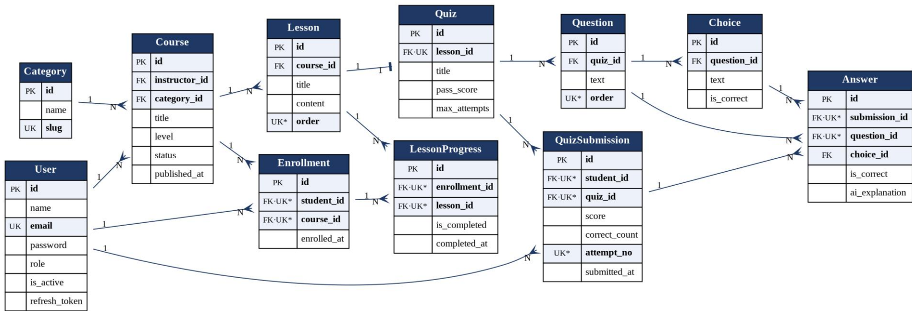
Hình 3.3. Sơ đồ quan hệ thực thể của hệ thống LearnQuiz
