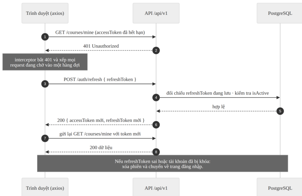
Hình 4.2. Biểu đồ tuần tự — tự động làm mới phiên đăng nhập
