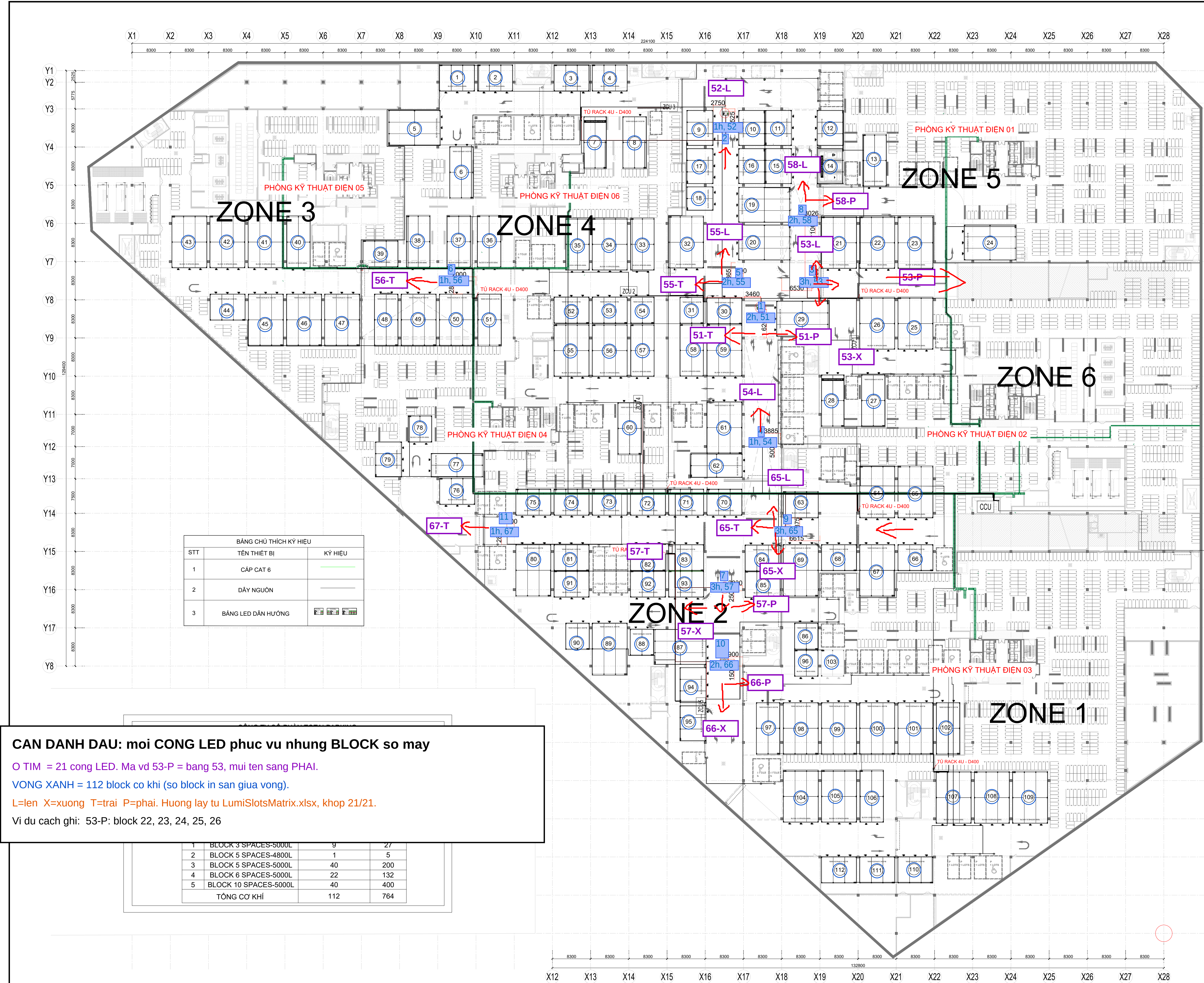
MẶT BẰNG TỔNG THỂ DÂY TÍN HIỆU TẦNG HẦM - CLUSTER 01
