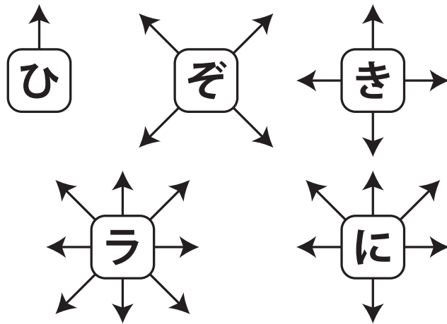
図 2 駒の動き
