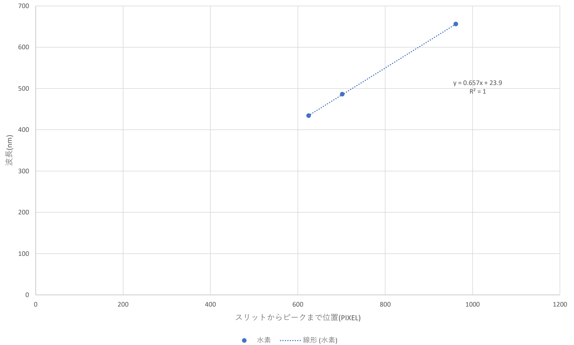
水素のスペクトルのピークと波長の関係
