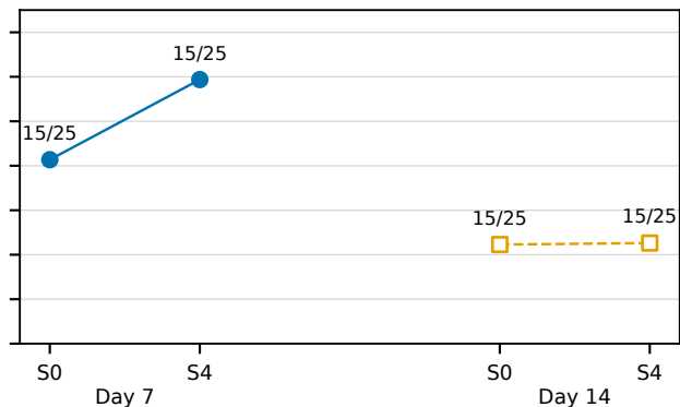
D F1
