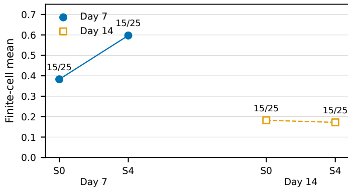
C CSI
