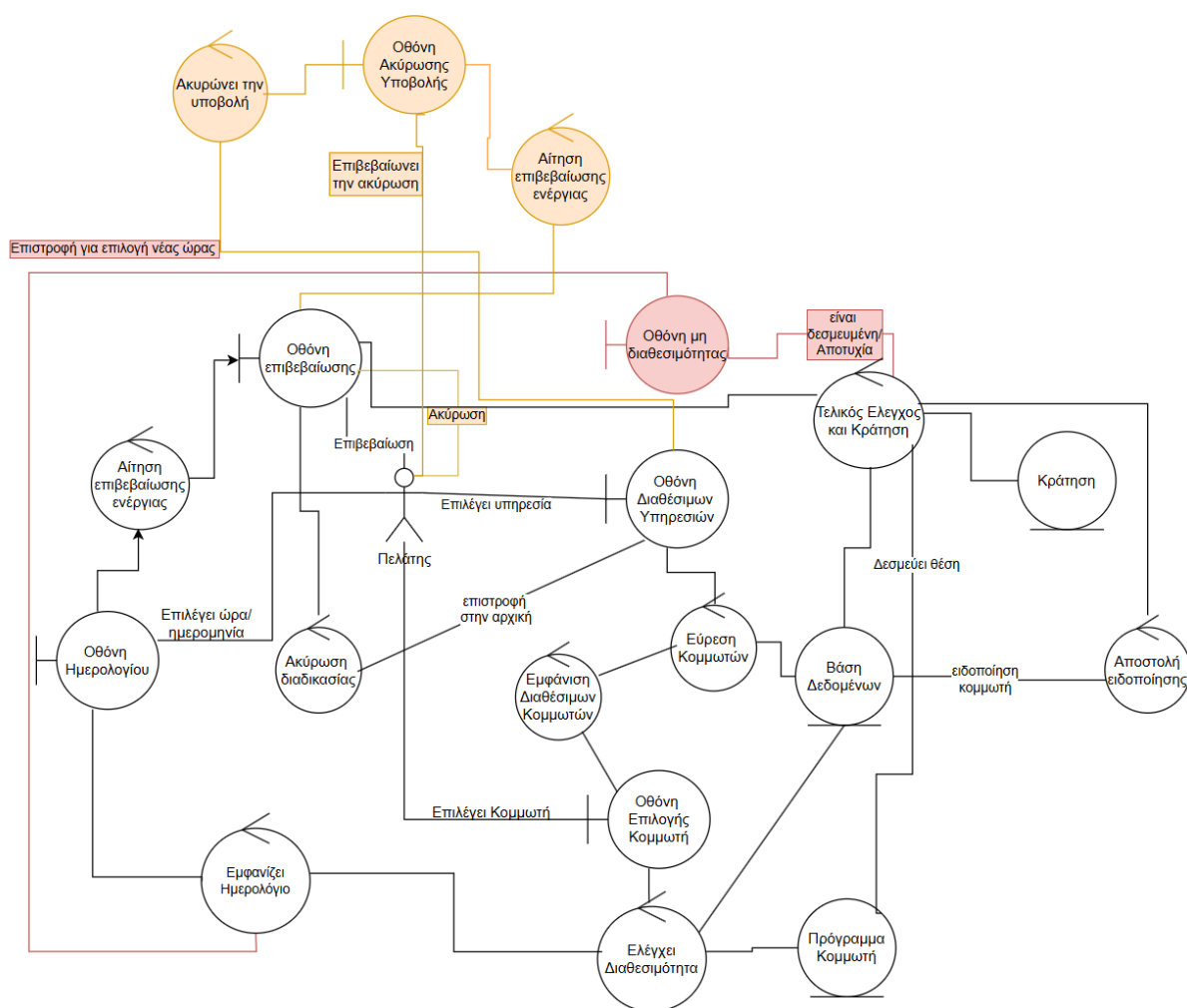
Σχήμα 4.2: Robustness diagram για την περίπτωση χρήσης "Προβολή Διαθέσιμων Ραντεβού & Κλείσιμο Ραντεβού"
