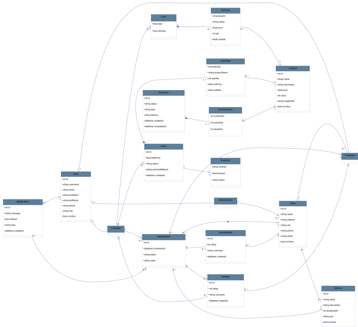
Σχήμα 3.1: Domain Model
