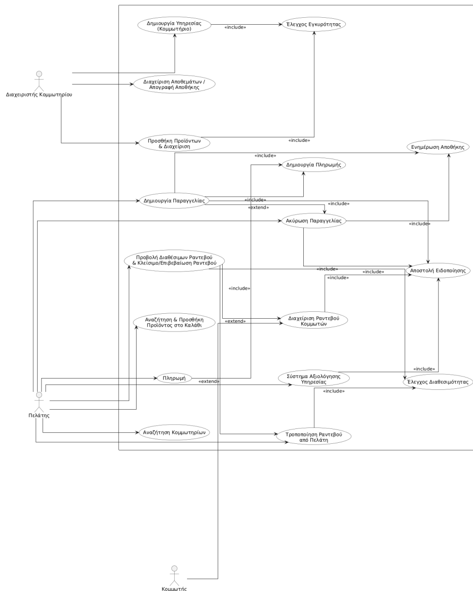
Σχήμα 2.1: Use-case διάγραμμα
