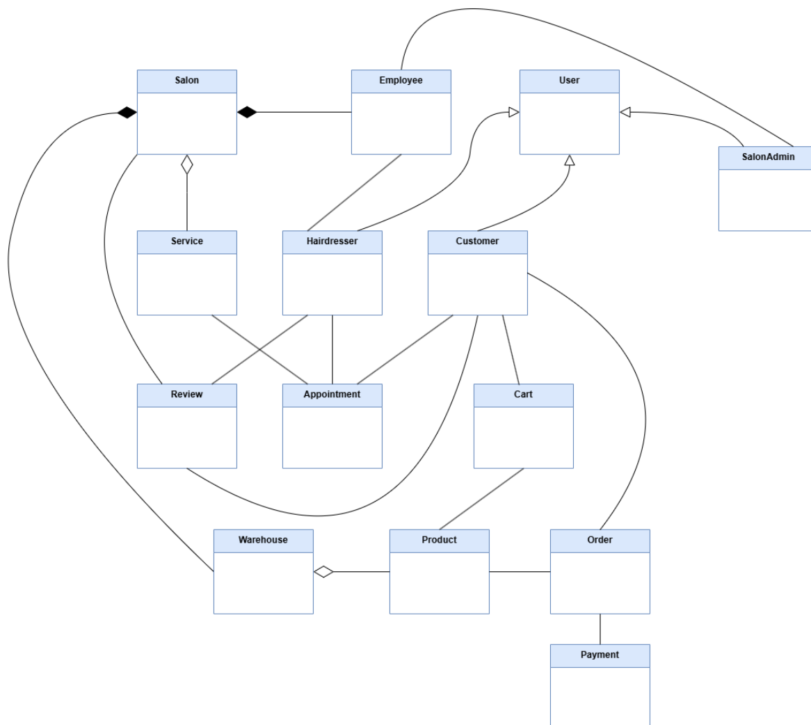
Σχήμα 3.1: Domain Model
