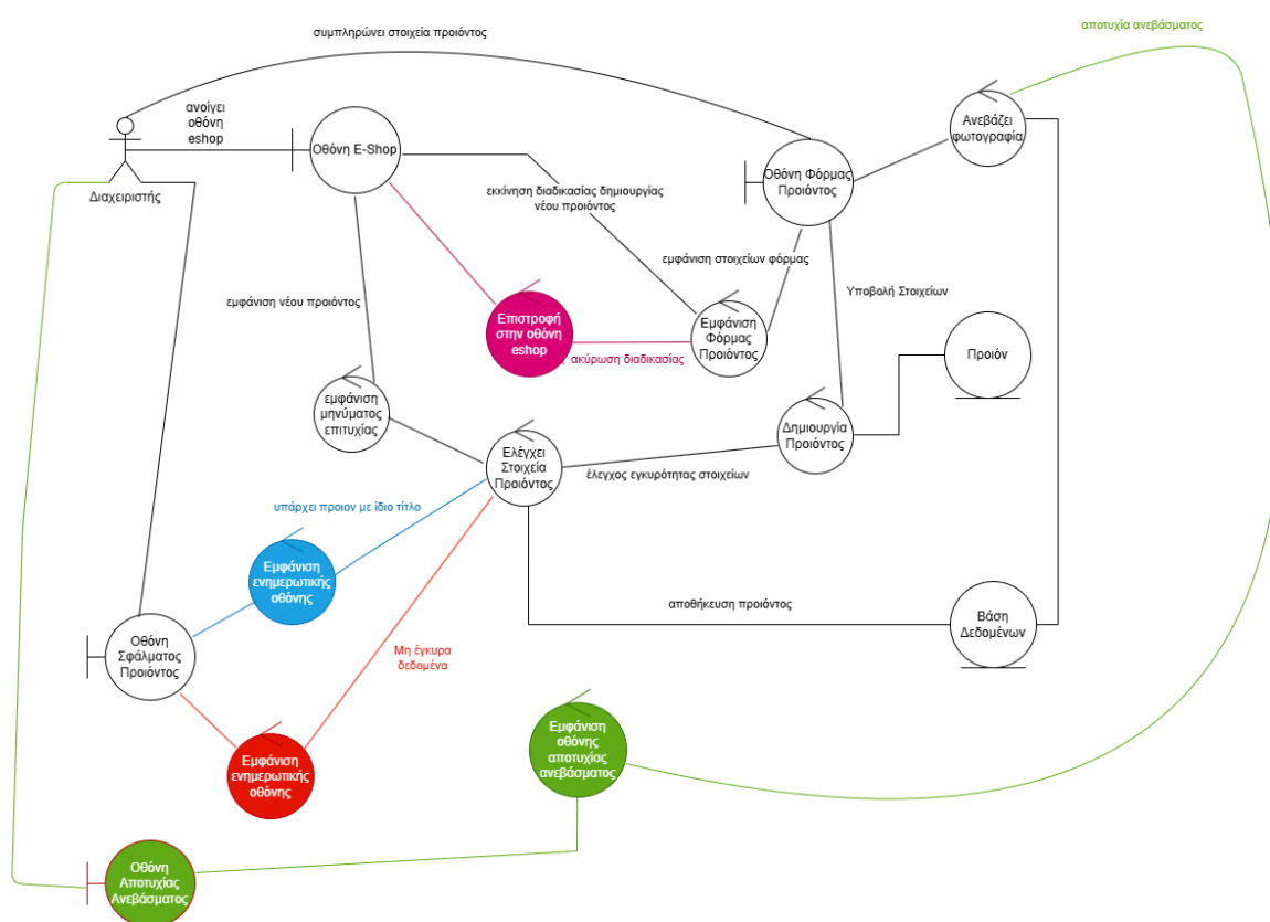
Σχήμα 4.8: Robustness diagram για την περίπτωση χρήσης "Προσθήκη Προϊόντων Διαχείριση"
