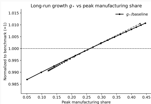
(b) g^*
