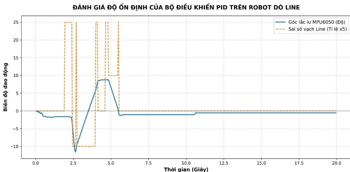
Hình 5.7: Đánh giá độ ổn định của robot khi dùng bộ điều khiển PID
