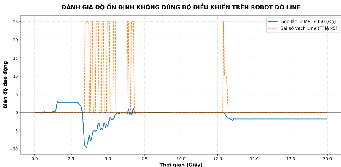
Hình 5.6: Đánh giá độ ổn định của robot khi không dùng bộ điều khiển PID
