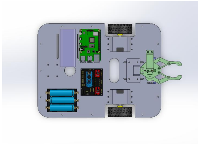
Hình 3.3: Bố trí các linh kiện phần đế robot (Kích thước 330mm x 250mm)
