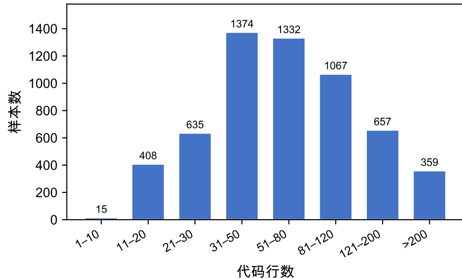
( a ) 代码行数分布
