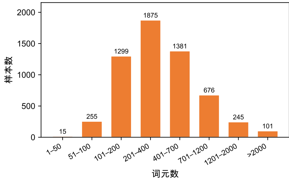
( b ) 词元数分布
