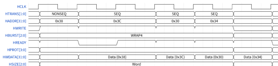
图 A.9 AHB 突发写传输
