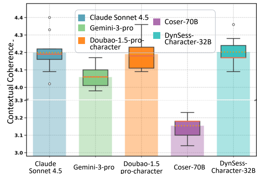
(d). Contextual Coherence.
