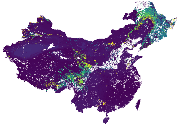
SSP585
