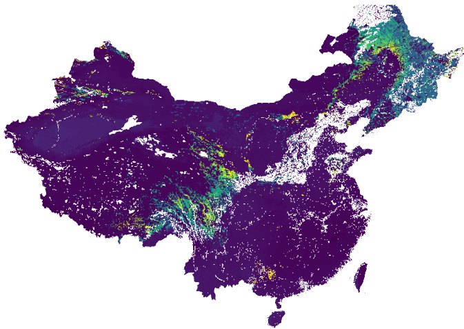
SSP245
