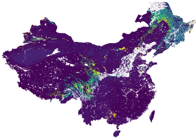
SSP126
