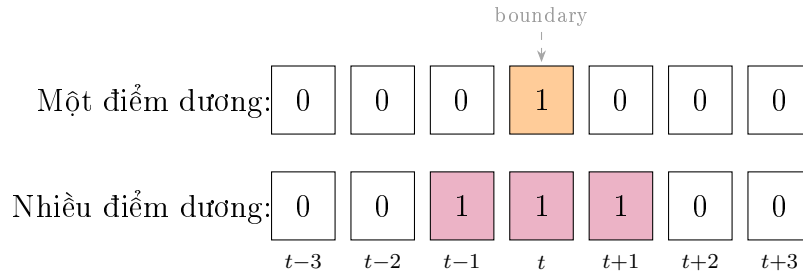
Hình 3.9: Minh họa nhãn một điểm dương (one-hot) và nhiều điểm dương (many-hot). Nhãn một điểm dương chỉ gán 1 tại đúng khung ranh giới t ; nhãn nhiều điểm dương mở rộng thêm t \pm 1 , cung cấp tín hiệu gradient dày đặc hơn quanh vùng ranh giới.
