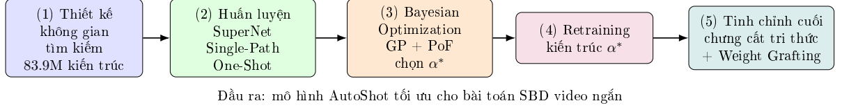
Hình 3.7: Sơ đồ 5 pha của quy trình NAS trong AutoShot: (1) Thiết kế không gian tìm kiếm với 83.9M kiến trúc; (2) Huấn luyện SuperNet theo chiến lược Single-Path One-Shot; (3) Tìm kiếm kiến trúc tối ưu bằng Bayesian Optimization (GP + PoF); (4) Huấn luyện lại kiến trúc \alpha^* ; (5) Tinh chỉnh bằng chưng cất tri thức và Weight Grafting.
