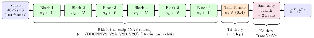
Hình 3.5: Sơ đồ tổng thể mô hình AutoShot gồm 7 vị trí kiến trúc cần tìm kiếm. Sáu vị trí đầu là các khối tích chập phân tách 3D chọn từ \mathcal{V} = \{\text{DDCNNV2}, \text{DDCNNV2A}, \text{DDCNNV2B}, \text{DDCNNV2C}\} với các siêu tham số (nc, nd) ; vị trí thứ 7 là khối Transformer 1D với số lớp tự chú ý \alpha_7 \in \{0, 1, 2, 3, 4\} . Nhánh similarity và hai đầu phân loại được kế thừa nguyên vẹn từ TransNetV2, do đó mọi cải thiện đo được đều quy về sự khác biệt ở 7 quyết định \alpha_1, \dots, \alpha_7 của NAS.
