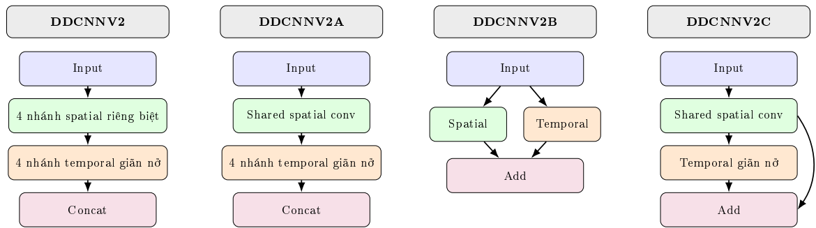
Hình 3.6: Bốn biến thể khối tích chập 3D phân tách trong không gian tìm kiếm của AutoShot. Từ trái qua phải: DDCNNV2 (spatial riêng biệt từng nhánh, concat), DDCNNV2A (shared spatial, concat), DDCNNV2B (spatial + temporal song song, cộng dồn theo P3D), DDCNNV2C (spatial truyền tuần tự vào temporal, cộng dồn). Tất cả đều dùng tích chập thời gian 1D giãn nở đa nhánh.
