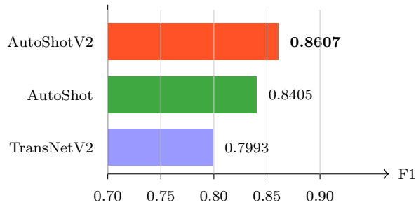
Hình 4.3: So sánh F1 giữa các mô hình trên tập SHOT (200 video kiểm tra). AutoShotV2 đạt F1 = 0.8607 theo lựa chọn tốt nhất trong giao thức so sánh chính, cải thiện +2.02 điểm phần trăm so với AutoShot tự chạy lại và +6.14 điểm phần trăm so với TransNetV2 mô hình cơ sở.
