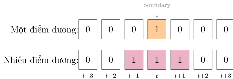
Hình 3.9: Minh họa nhãn một điểm dương và nhãn nhiều điểm dương. Nhãn một điểm dương chỉ gán 1 tại đúng khung ranh giới t ; nhãn nhiều điểm dương mở rộng thêm t \pm 1 , cung cấp tín hiệu gradient dày đặc hơn quanh vùng ranh giới.
