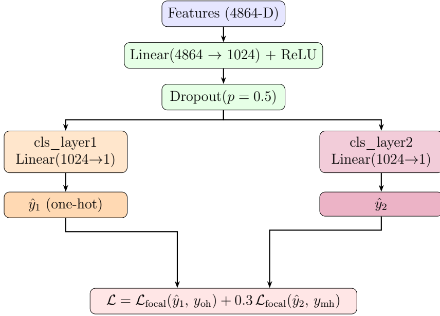
Hình 3.8: Kiến trúc tầng phân loại trong AutoShotV2. Tầng phân loại này nhận đặc trưng 4864-D từ mạng xương sống đã đóng băng và sinh hai đầu ra song song: nhánh một điểm dương định vị ranh giới chính xác và nhánh nhiều điểm dương học ngữ cảnh vùng biên.
